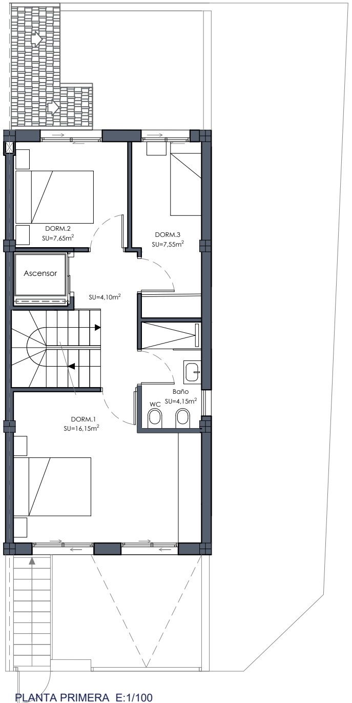
PLANTA PRIMERA E:1/100
