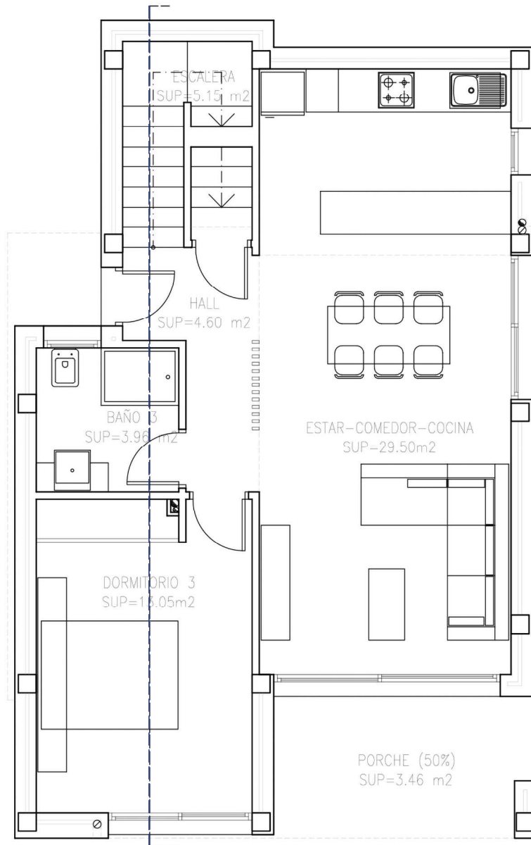
PLANTA BAJA - OPCIÓN A
