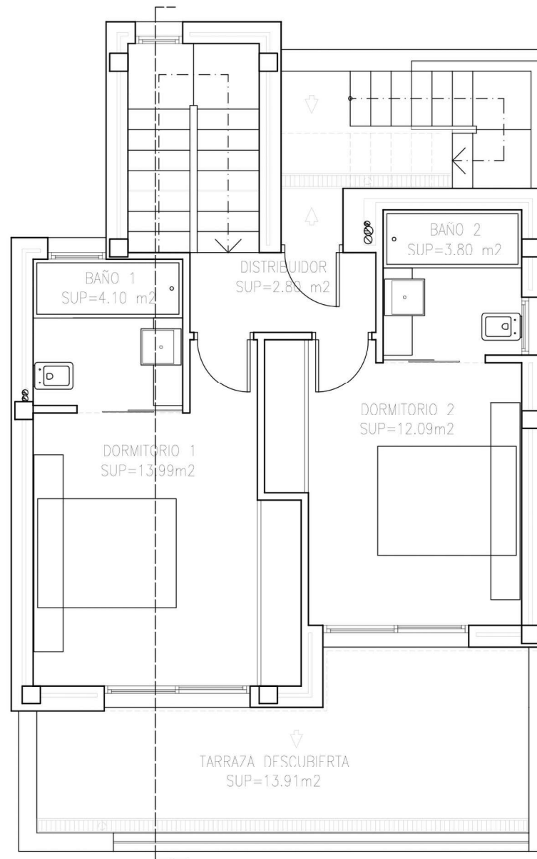
PRIMERA PLANTA
