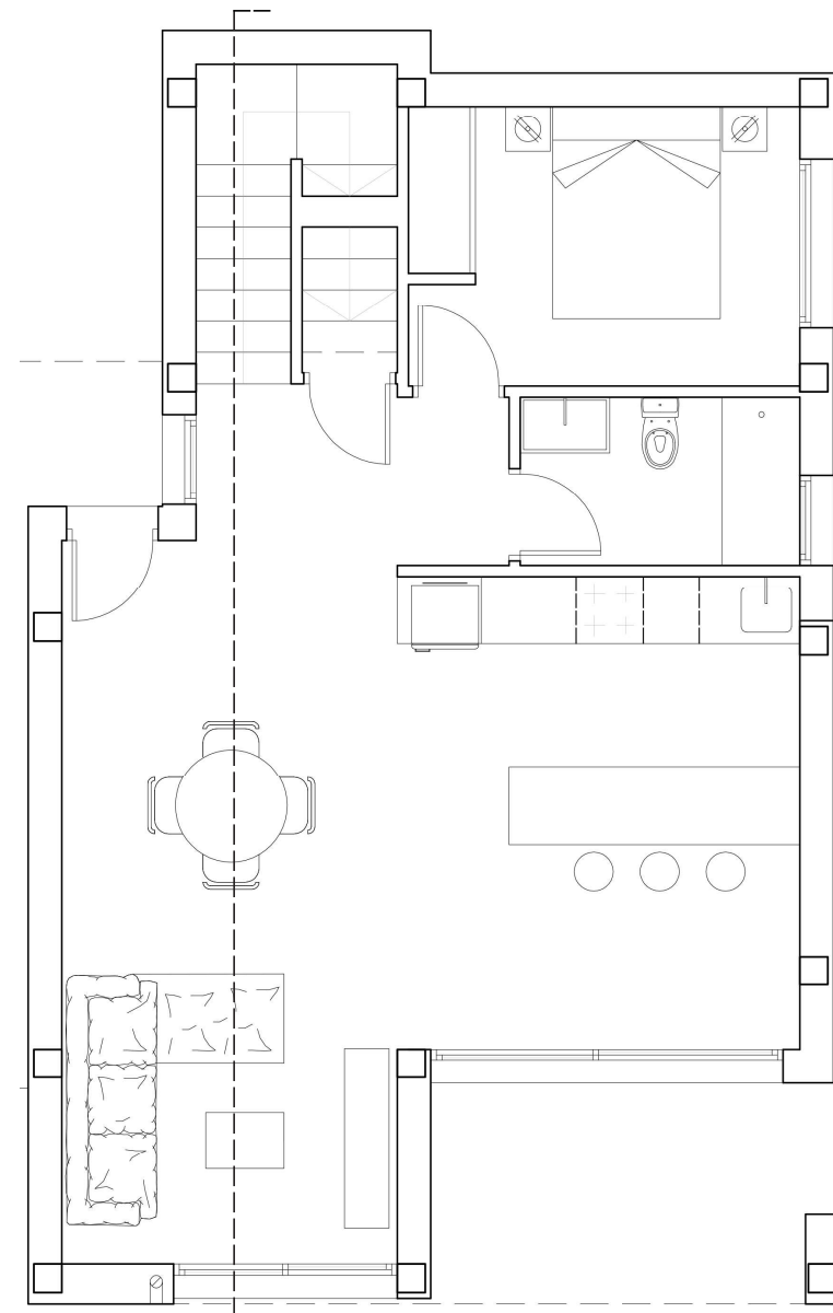
PLANTA BAJA - OPCIÓN B
