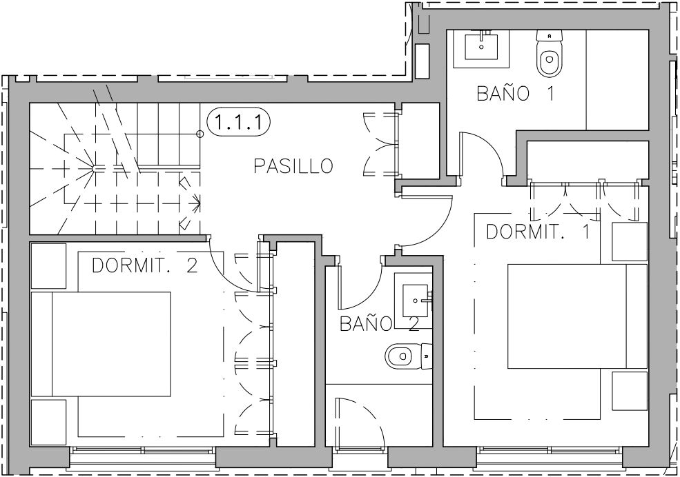
PLANTA 0
