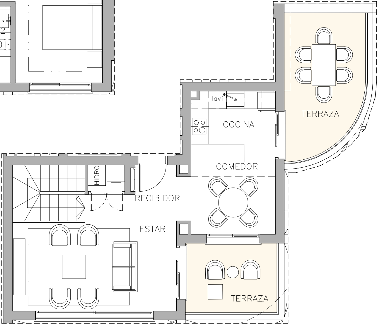
PLANTA PRIMERA
