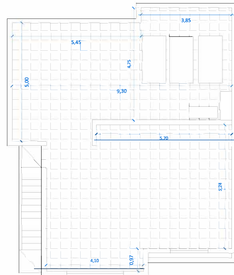
SOLARIUM MODELO A
