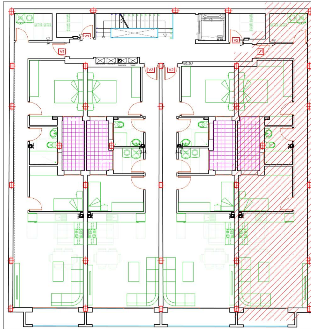
PRIMERA PLANTA
